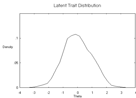
Fig. 5: Latent Trait Distribution
